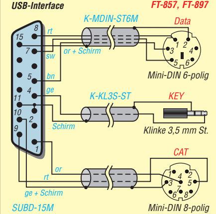
Bild A2-2: Verbindungskabel für den FT-100, -817, -857, -897
