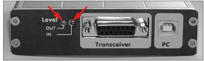
Bild 23: Rückansicht des Mustergerätes; der linke Pegelsteller ist für Modulation, der rechte für Empfangssignalpegel, rechtsherum bedeutet mehr Pegel.
